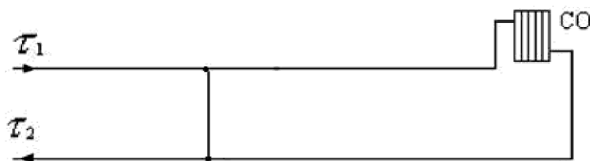
Рисунок 1.3.16.4 - Схема подключения потребителей к двухтрубной системе теплоснабжения
